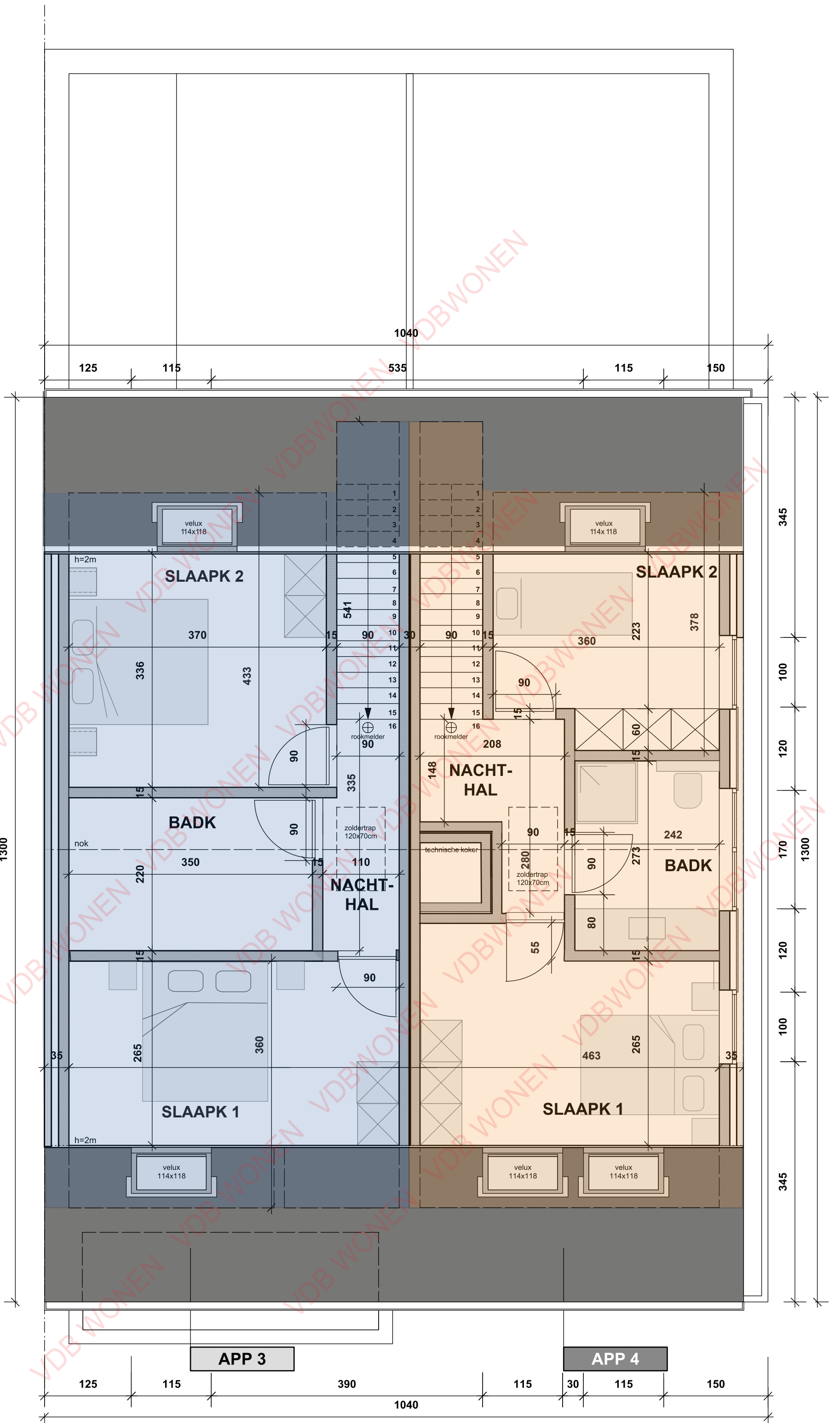
2° VERDIEPINGSPLAN (app.3&4)
